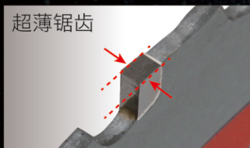
金属陶瓷材料锯齿
